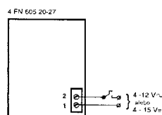
obr.2: zapojení přívodních vodičů na svorkovnice zvonků
