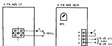
obr.2: zapojení přívodních vodičů na svorkovnice zvonků
