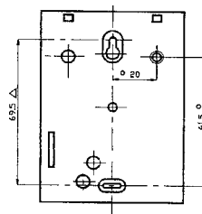
obr.1: spodní pohled na základní desku s rozmístěním upevňovacích otvorů
