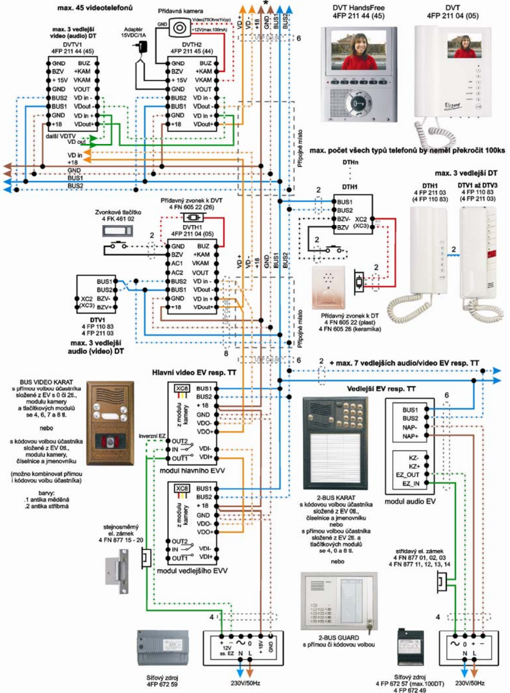
Obr. 3 Schéma zapojení videosystému
